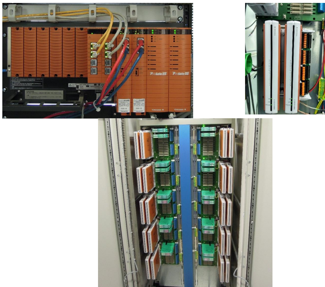
Рисунок 1 - Общий вид ИВК
