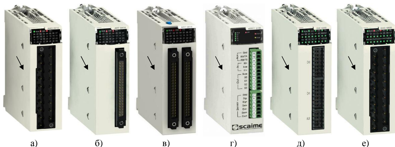
Рисунок 1 - Внешний вид модулей а) ВМХАМxxxxxy и ВМЕАНxxxxxy, б) ВМХАRТ0414у, в) ВМХАRТ0814у, г) РМЕSWT0100, д) ВМХЕНС0200у, е) ВМХЕНС0800у (x - цифра, y - пробел или символ «Н», образующие обозначение конкретного модуля)
