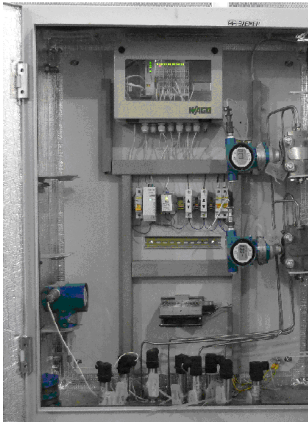
Рисунок 6 - Шкаф ШД3
