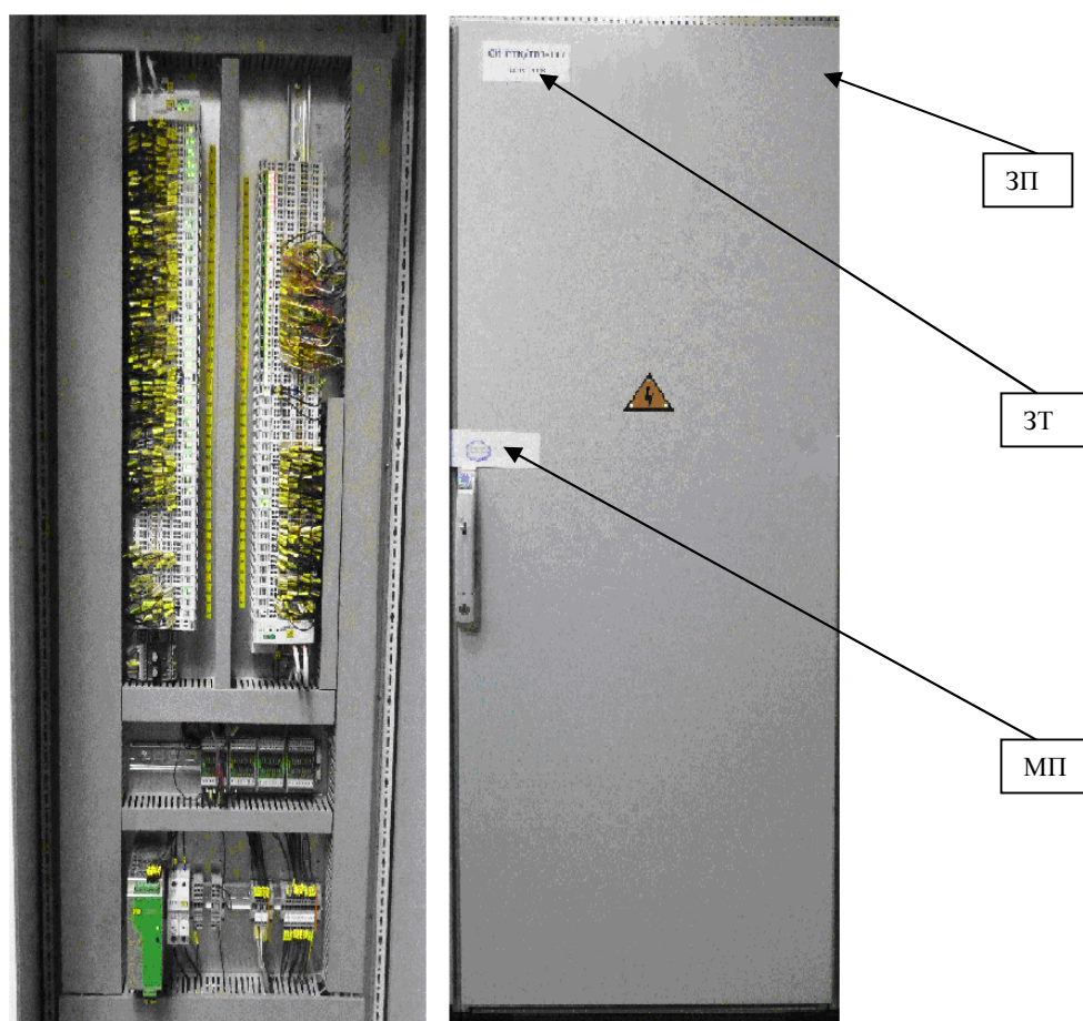
Рисунок 3 - Шкаф ШК ПКТ
