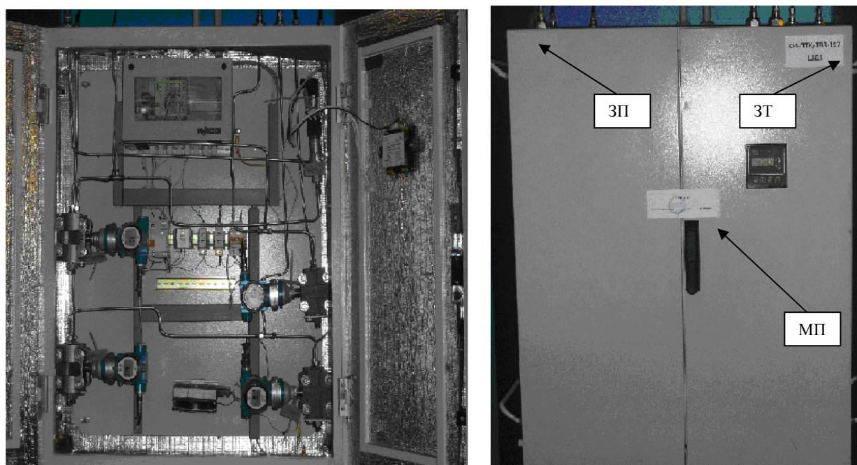
Рисунок 4 - Шкаф ШД1
