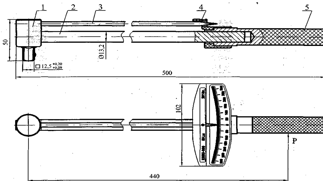
Рисунок 2 - Общий вид ключей моментных показывающих КМ-200
