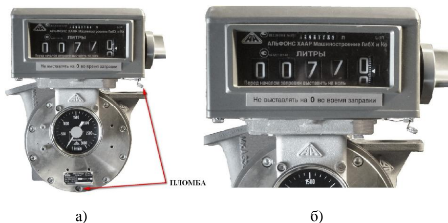
Рисунок 1 - Счетчик жидкости лопастной МКА
