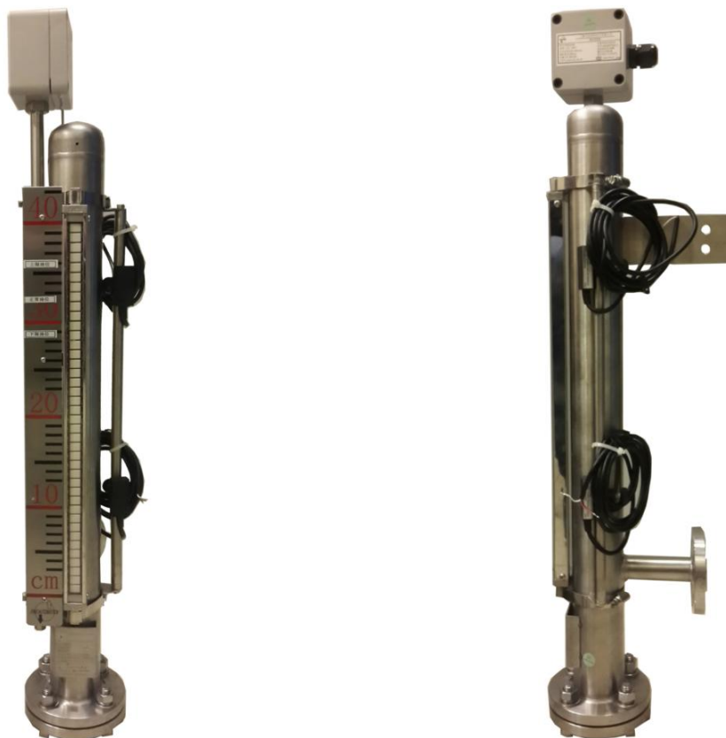
Рисунок 1 - Общий вид уровнемеров байпасных EF311A1H1I2-0400GM
