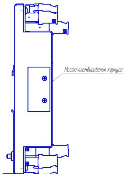
Рисунок 2 – Схема пломбировки контроллера от несанкционированного доступа
