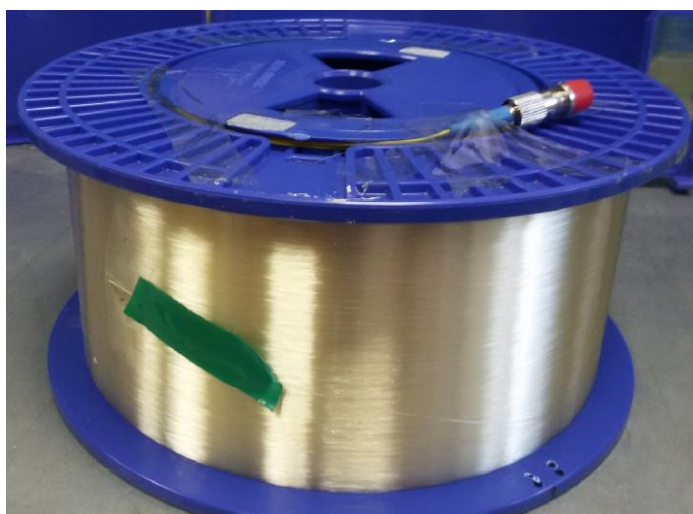
Рисунок 3 - Общий вид волоконно-оптических кабелей для систем мониторинга распределения температуры волоконно-оптических модульных повышенной дальности DTSXL
