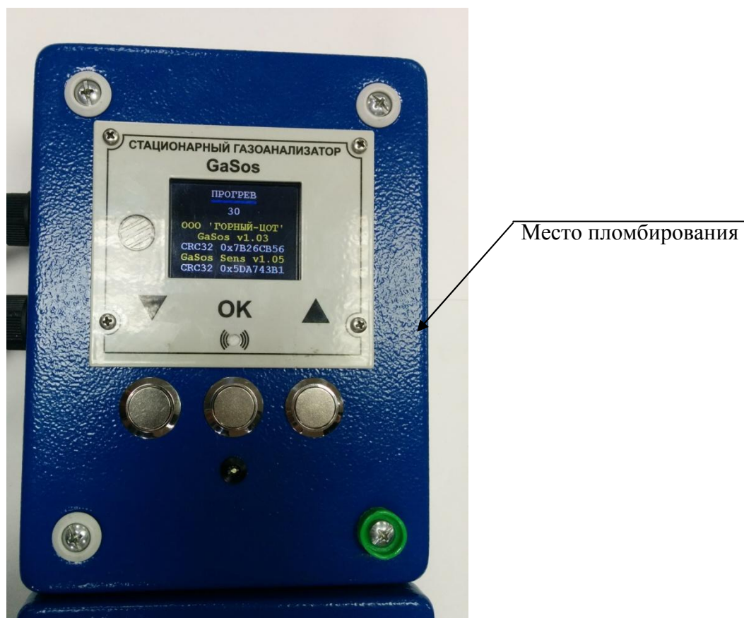
Рисунок 3 – Схема пломбирования корпуса блока измерения и индикации GaSos.M2-DD от несанкционированного доступа
