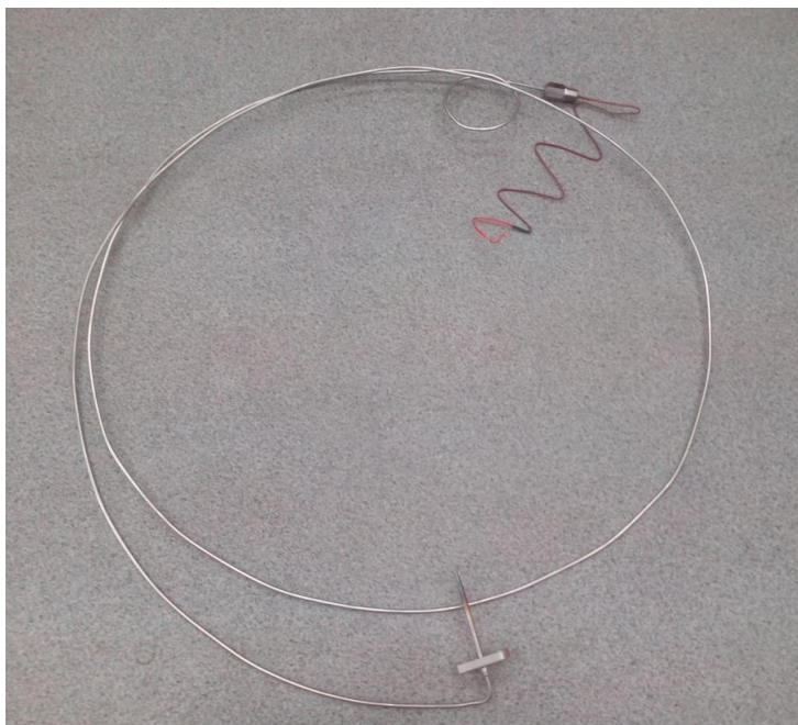
Рисунок 1 - Общий вид преобразователей термоэлектрических модели 361257-100
