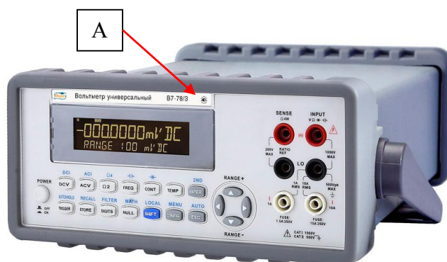
Рисунок 3 - Внешний вид вольтметров В7-78/3 и место нанесения знака утверждения типа (А)
