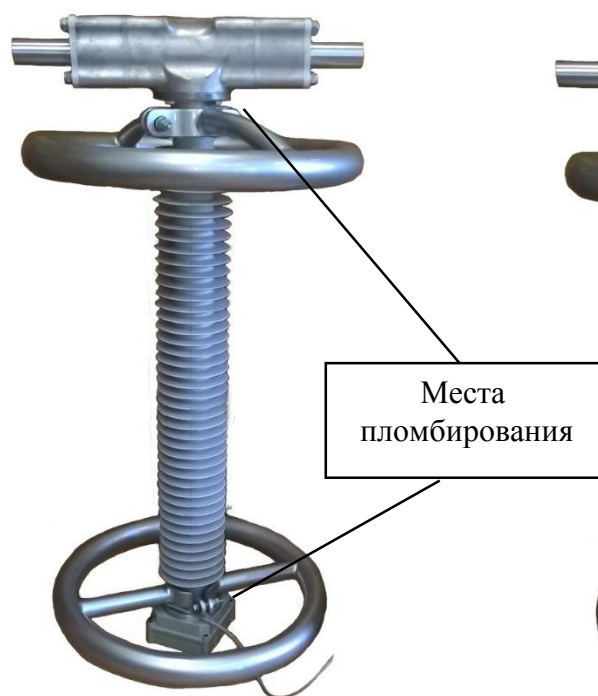
Рисунок 4 - Внешний вид исполнения ЦТТН 35 - 220 кВ опорного исполнения с электронными блоками в голове и основании колонны
