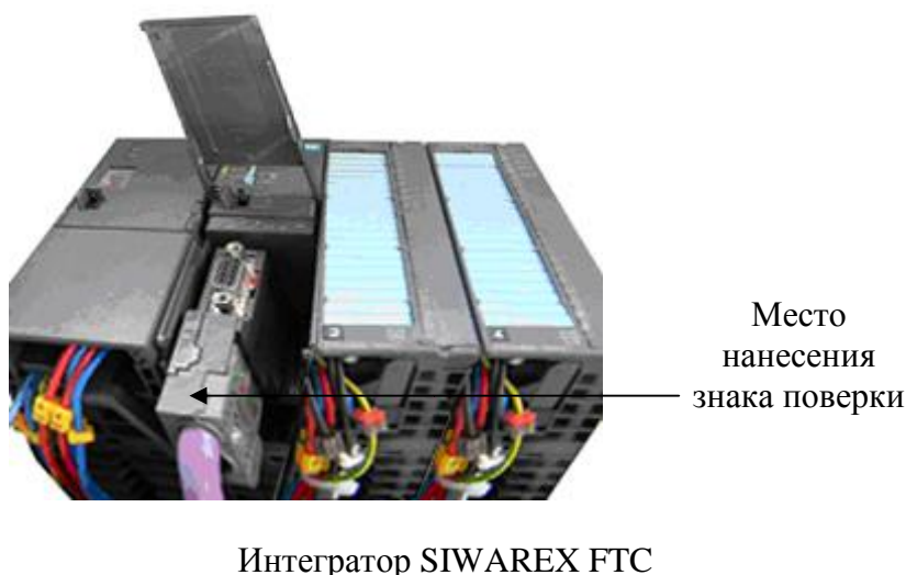
Рисунок 3 - Схемы пломбировки от несанкционированного доступа, обозначение места нанесения знака поверки на интеграторы ПВ-15 и SIWAREX FTC
