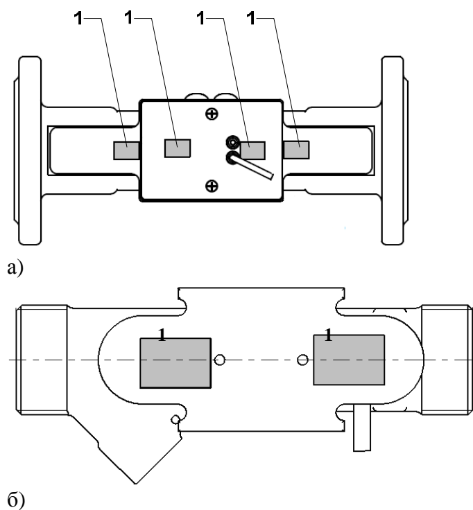
Рисунок 2 - Места пломбировки преобразователей ультразвуковых SonoSensor 30 а)- для фланцевого исполнения б)- для резьбового исполнения
