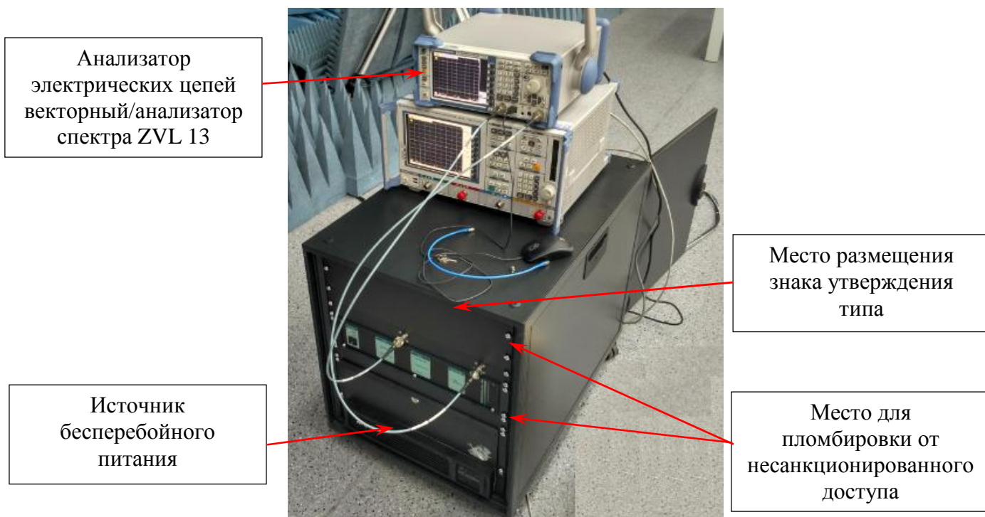
Рисунок 4 - Внешний вид приборной стойки для размещения элементов комплекса и места размещения знака утверждения типа
