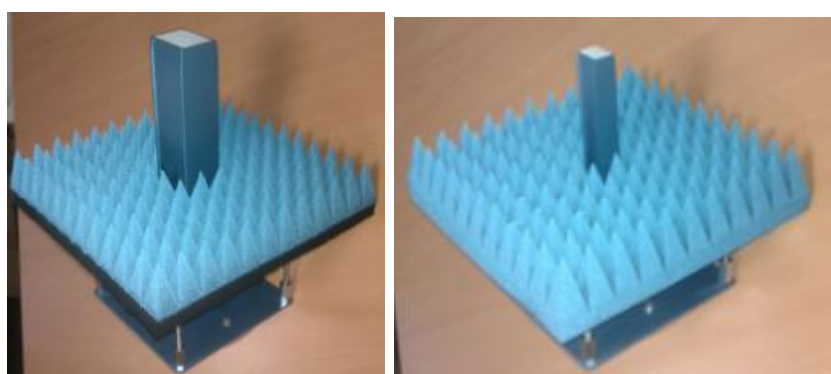
Рисунок 3 - Внешний вид антенны-зонда ТМАЗ 4-8 И диапазона частот 4 - 8 ГГц (слева), внешний вид антенны-зонда ТМАЗ 8-18 И диапазона частот 8 - 18 ГГц (справа)
