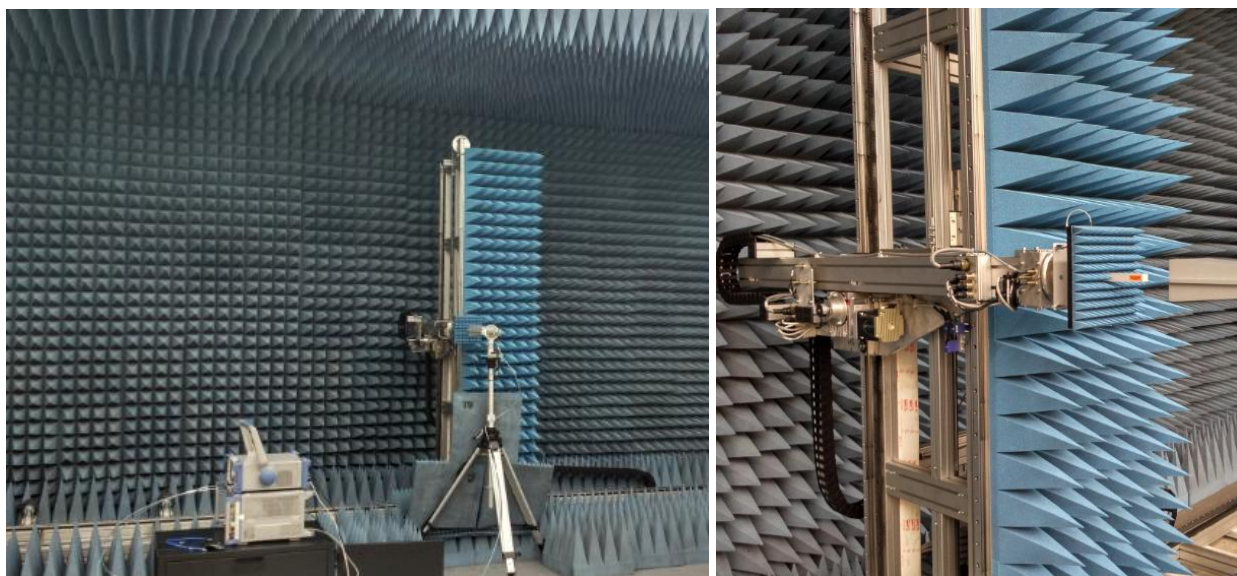
Рисунок 1 - Общий вид конструкции сканера ТМП 04П 9.0 x 2.25
