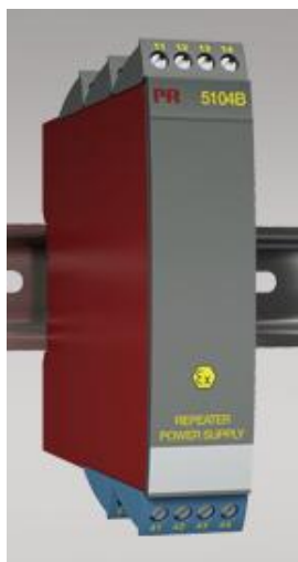
Рисунок 5 - Общий вид преобразователей измерительных серии PR модификаций 5104, 5105, 5106, 5107, 5114, 5115, 5131, 5116, 5223
