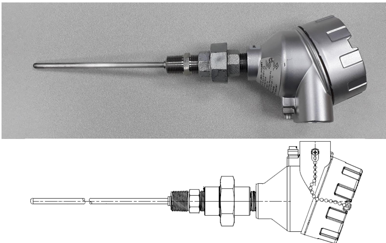
Рисунок 1 - Общий вид преобразователей термоэлектрических модели 111Т0537Р0001
