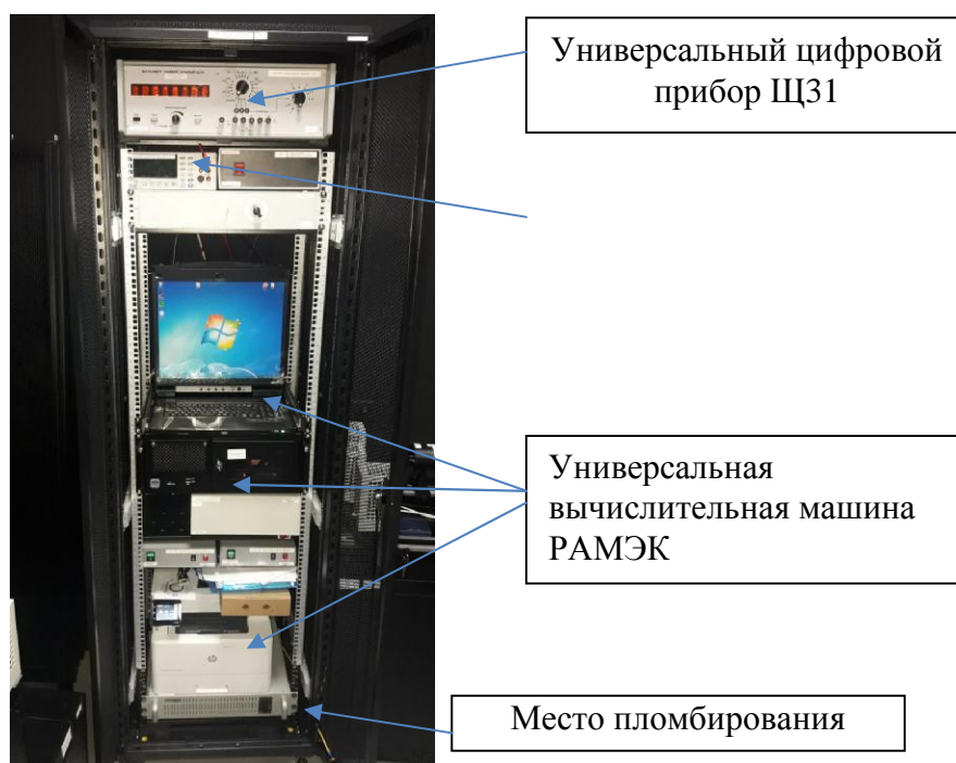
Рисунок 2 - Общий вид и схема пломбировки от несанкционированного доступа устройства управления, хранения и обработки измерительной информации комплекта аппаратуры
