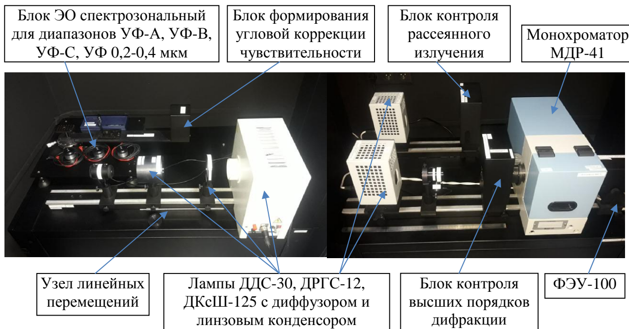
Рисунок 1 - Общий вид компаратора единицы ЭО из состава комплекта аппаратуры
