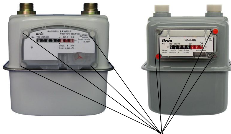
Места пломбирования
