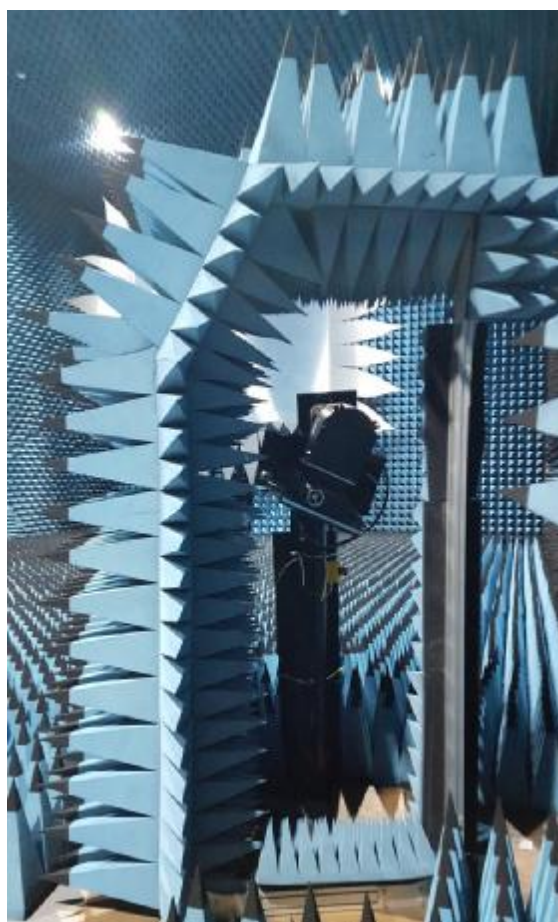
Рисунок 3 - Внешний вид ОПУ облучателя зеркала радиоколлиматора и его укрытия
