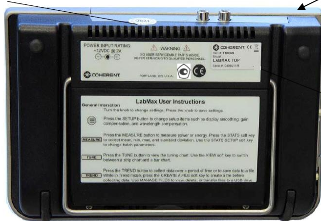
Рисунок 2 – Схема пломбировки от несанкционированного доступа и место нанесения знака поверки.
