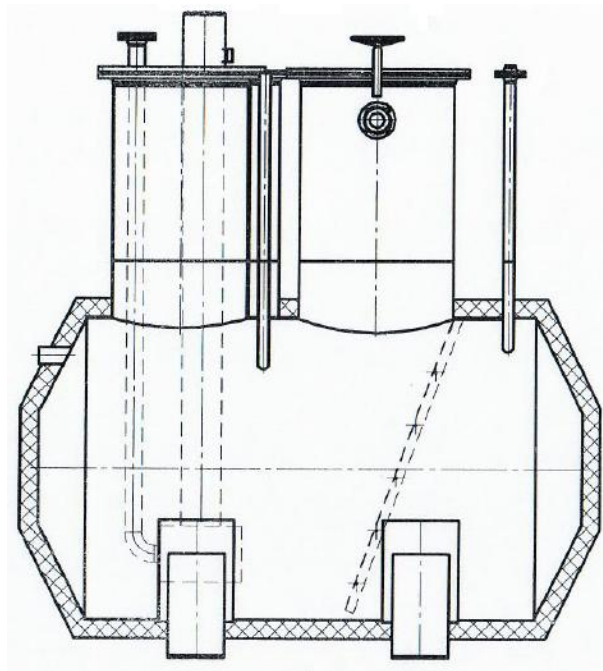
Рисунок 1 - Общий вид резервуаров стальных горизонтальных цилиндрических РГС-5
