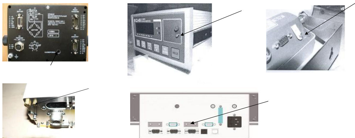
Рисунок 3 - Места пломбирования приборов весоизмерительных
