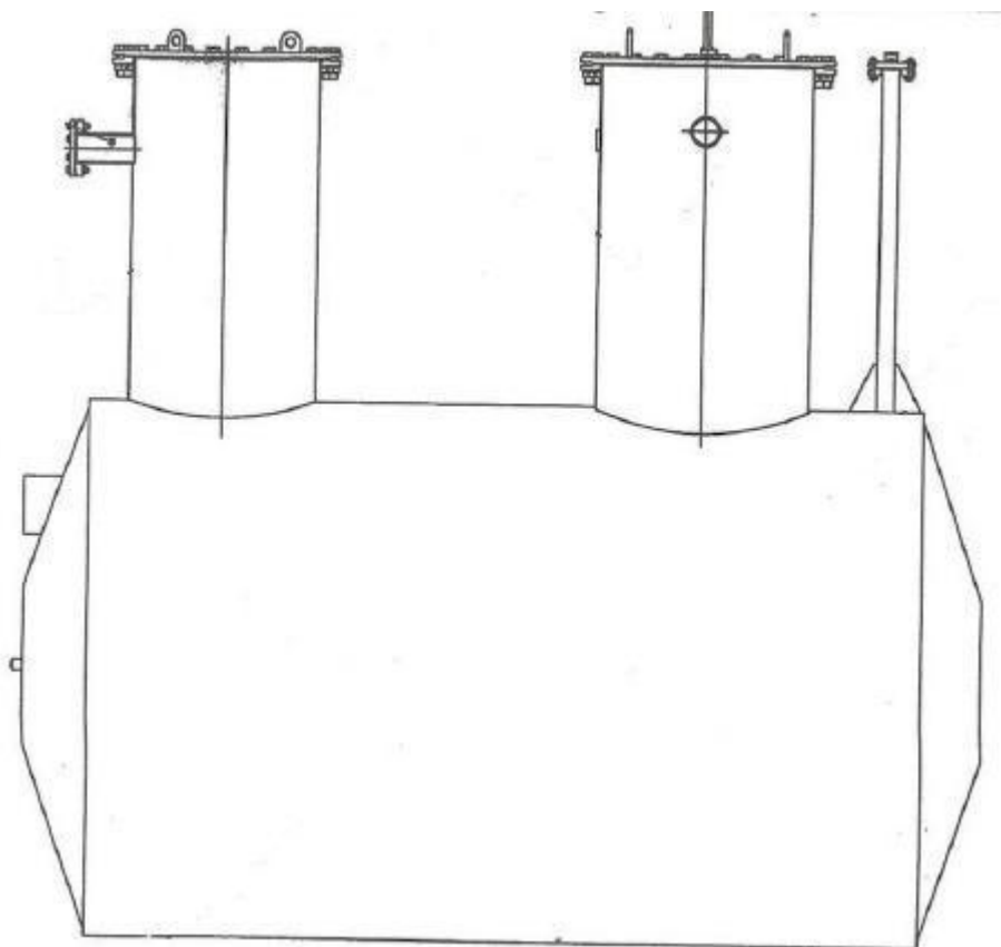
Рисунок 1 - Эскиз резервуара РГС-16
