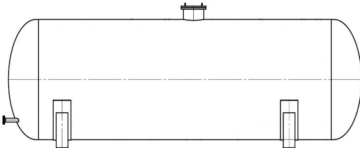
Рисунок 1 - Общий вид резервуара стального горизонтального цилиндрического РГС-200
