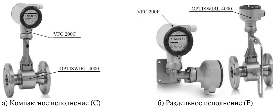
Рисунок 1 – Общий вид расходомеров-счетчиков вихревых OPTISWIRL 4200.
