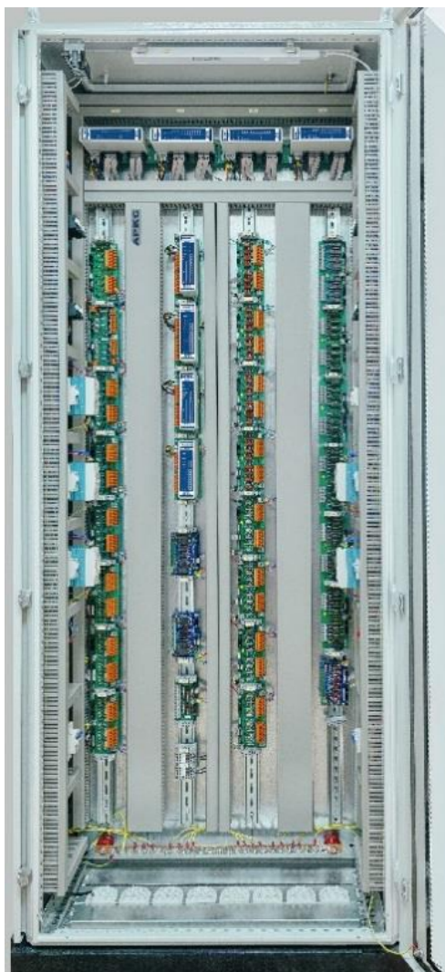
Рисунок 1 - Контроллерный шкаф мульти-платформенной системы «МИРТС»
