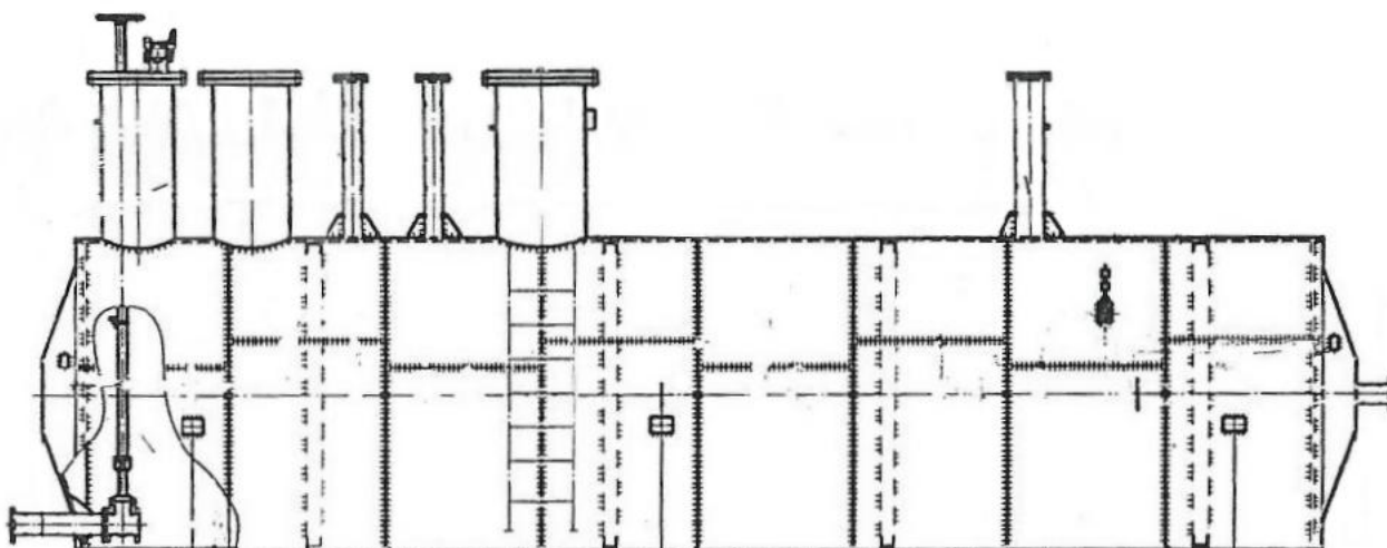
Рисунок 1 - Эскиз резервуаров РГСП-100
