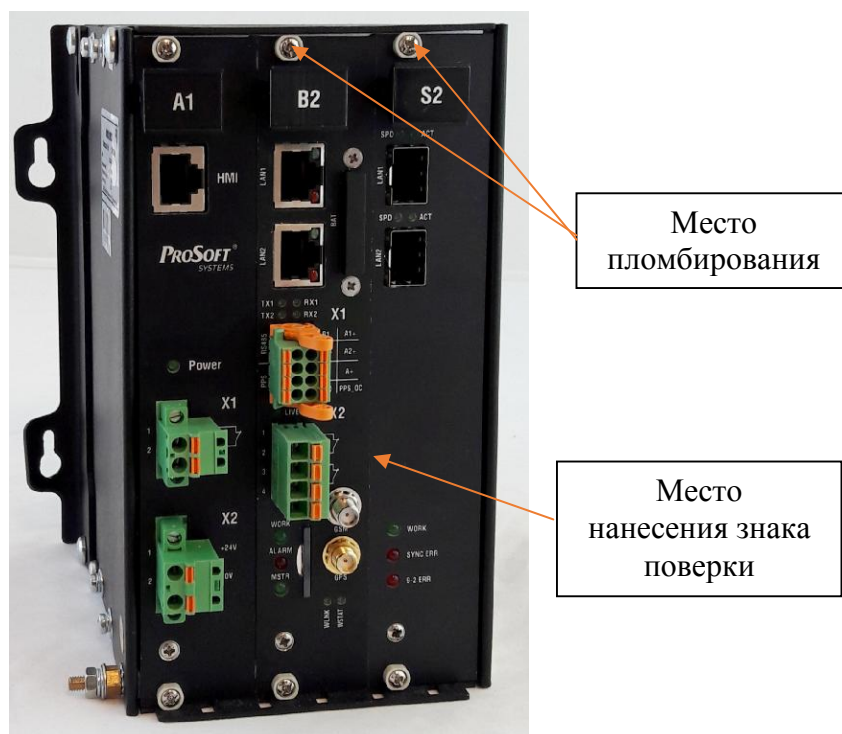
Рисунок 6 – Места пломбирования и нанесения знака проверки
