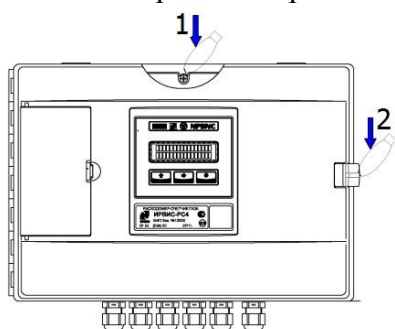
д) блок интерфейса и питания (корпусное исполнение)
