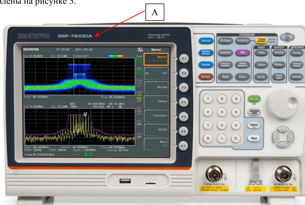
Рисунок 1 – Общий вид анализаторов GSP-79330A и место нанесения знака утверждения типа (А)
