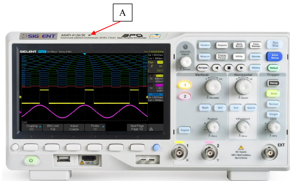
Рисунок 1 – Общий вид осциллографов и место нанесения знака утверждения типа (А)
