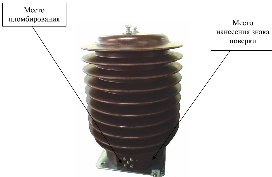
Рисунок 1 - Общий вид трансформаторов тока SMTSM-38 с указанием мест пломбирования от несанкционированного доступа и нанесения знака поверки
