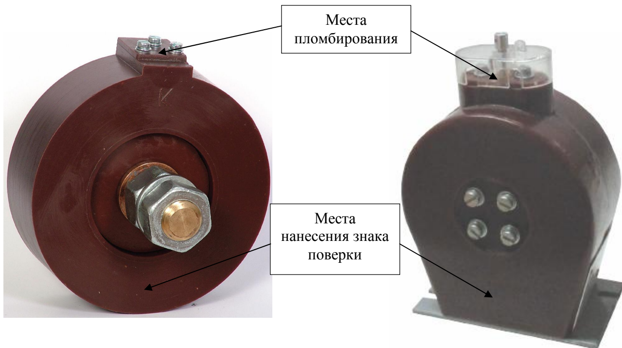
в) трансформаторы ST-3,6
