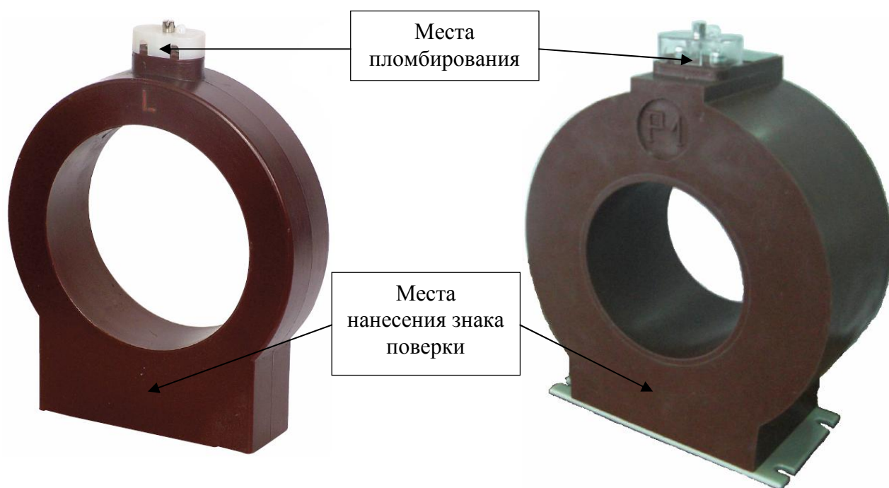
а) трансформаторы ST-081 А, ST-081 В и ST-081 С
