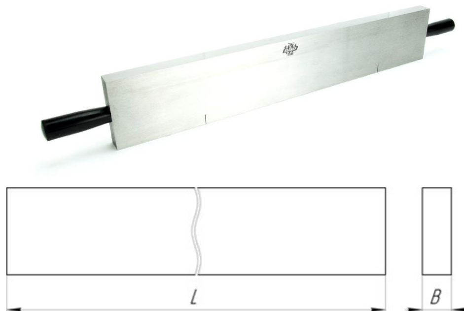
Рисунок 1 – Общий вид брусков модели 1 и обозначение их основных размеров
