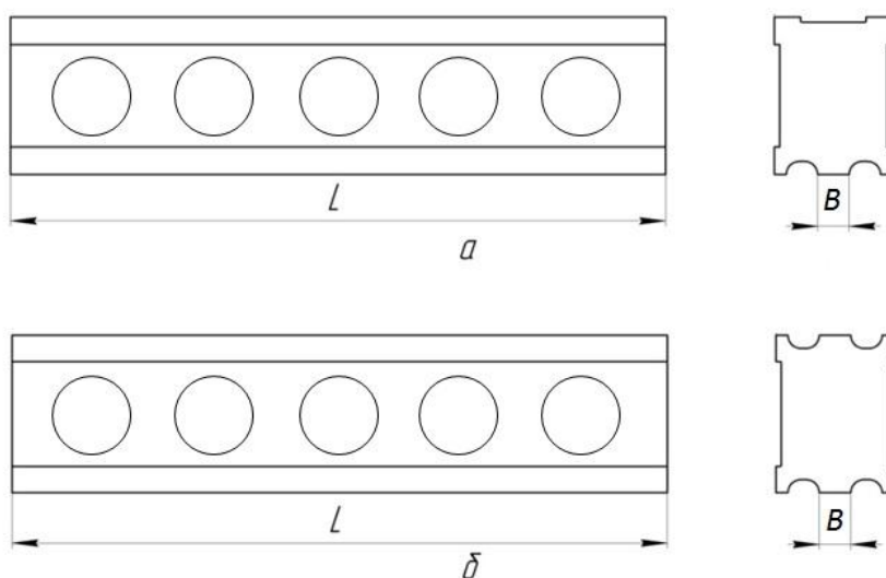
Рисунок 8 - Общий вид брусков модели 8 и обозначение их основных размеров а – с одной рабочей поверхностью; б – с двумя рабочими поверхностями
