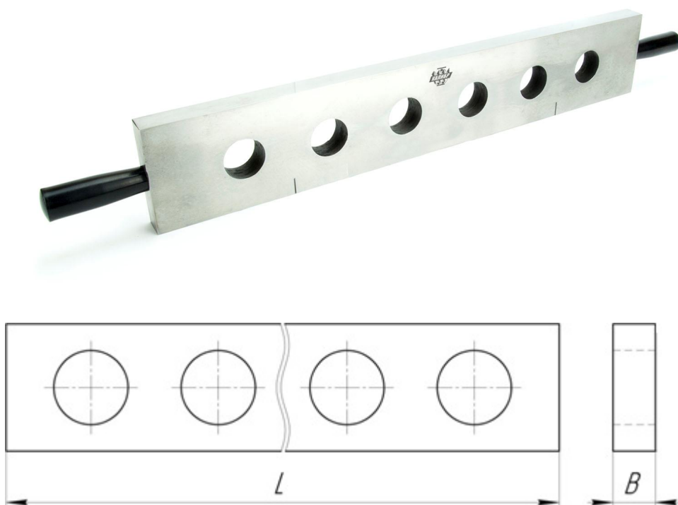
Рисунок 2 - Общий вид брусков модели 2 и обозначение их основных размеров
