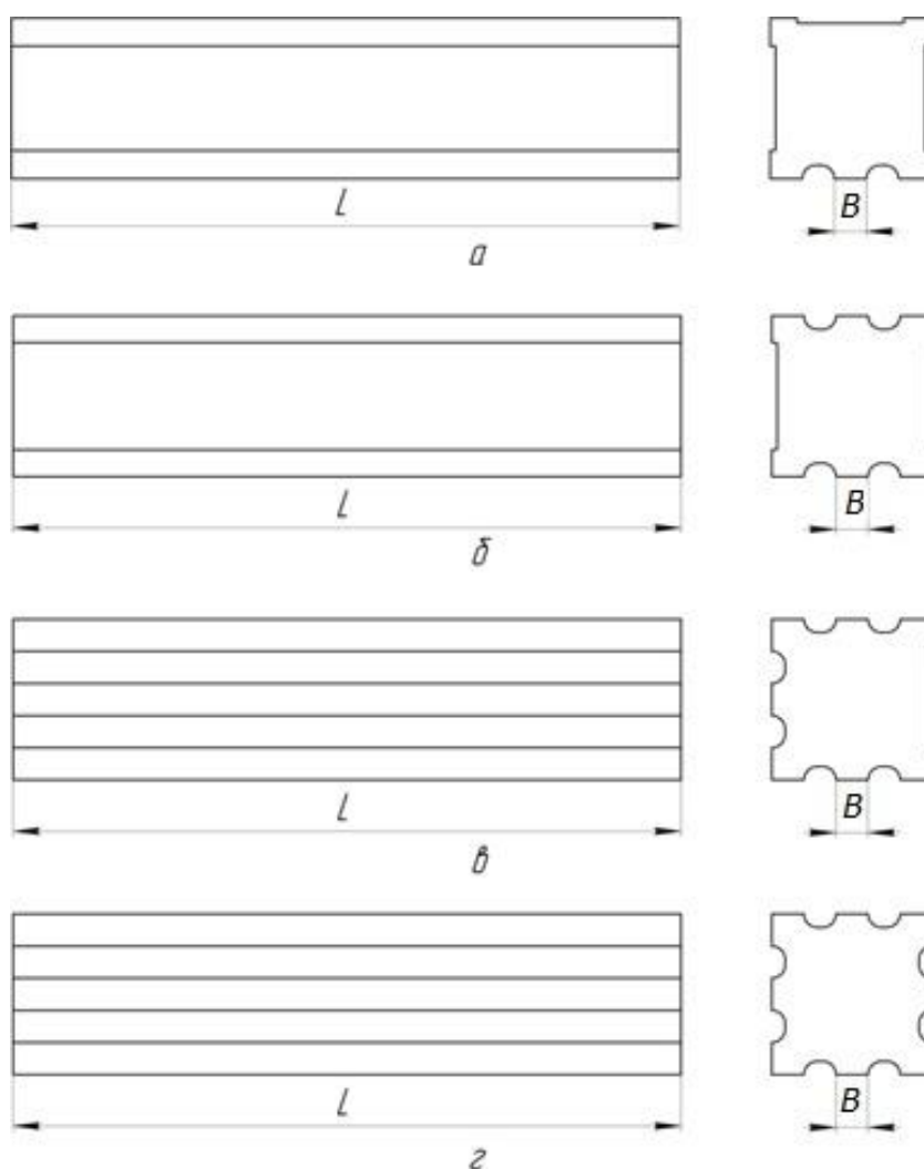
Рисунок 5 - Общий вид брусков модели 5 и обозначение их основных размеров а – с одной рабочей поверхностью; б – с двумя рабочими поверхностями; в – с тремя рабочими поверхностями; г – с четырьмя рабочими поверхностями.
