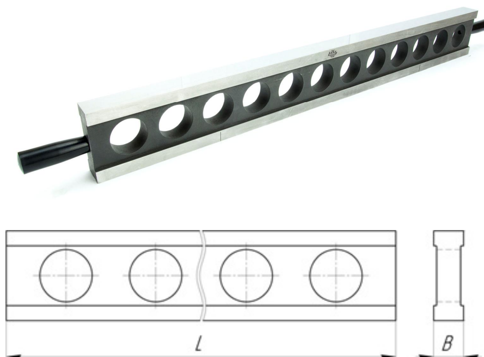
Рисунок 4 - Общий вид брусков модели 4 и обозначение их основных размеров
