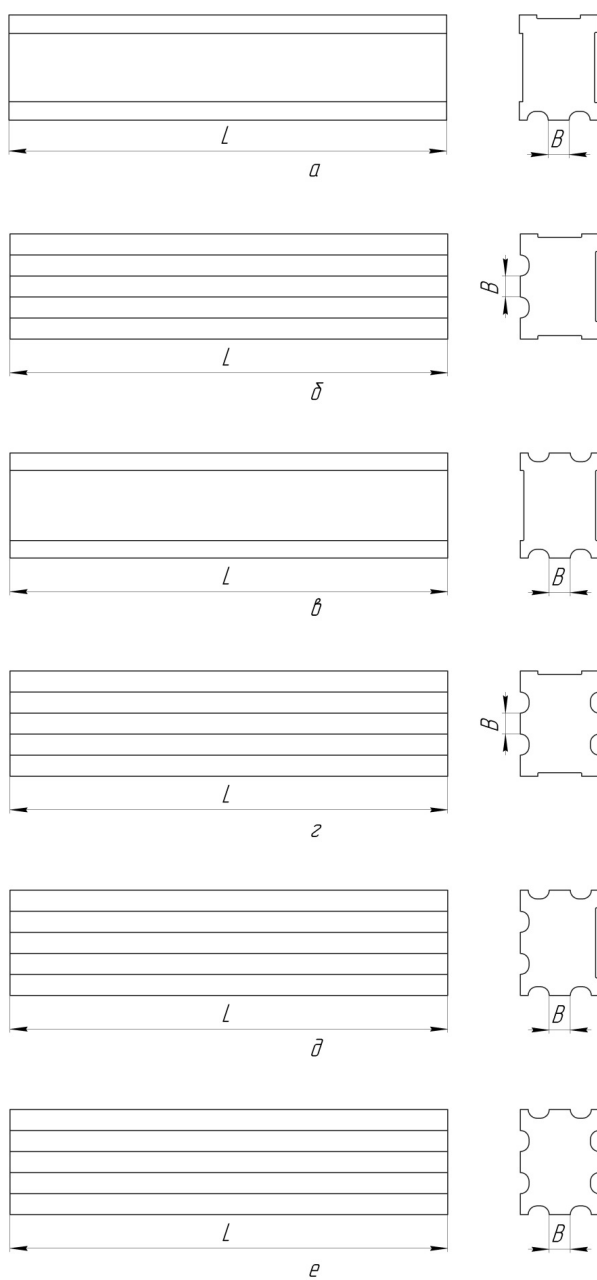
Рисунок 7 - Общий вид брусков модели 7 и обозначение их основных размеров а, б – с одной рабочей поверхностью; в, г – с двумя рабочими поверхностями; д – с тремя рабочими поверхностями; е – с четырьмя рабочими поверхностями.
