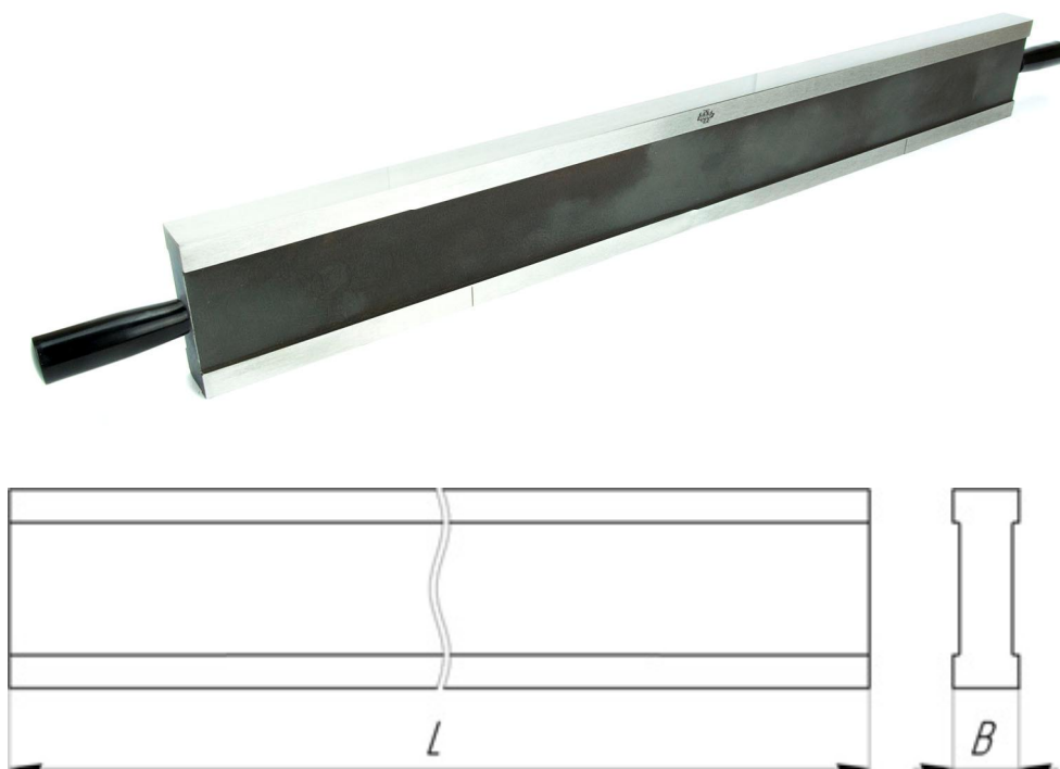
Рисунок 3 - Общий вид брусков модели 3 и обозначение их основных размеров
