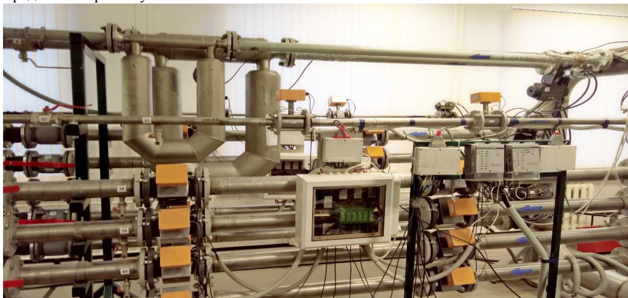
Рисунок 1 – Общий вид установки поверочной СПРУТ 200М
