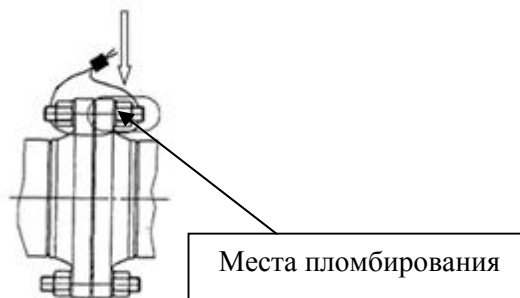
Рисунок 2 – Схема пломбировки от несанкционированного доступа, обозначение места нанесения знаков поверки на фланцевые соединения расходомеров установки поверочной СПРУТ 200М
