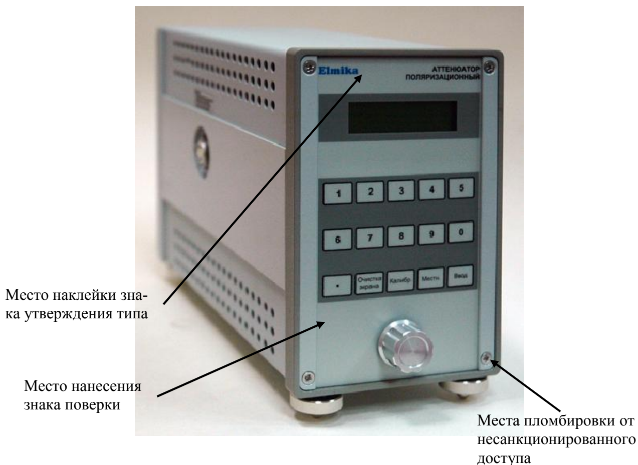
Рисунок 1 - Общий вид аттенюаторов моделей АП-19М, АП-20М, АП-21М, АП-22М, АП-32М, АП-35М
