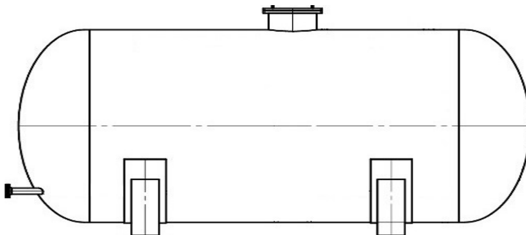
Рисунок 1 – Эскиз резервуаров стальных горизонтальных цилиндрических РГС-25
