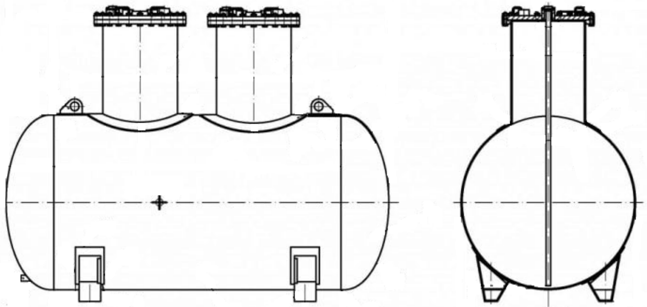
Рисунок 1 – Эскиз резервуара РГС-12,5
