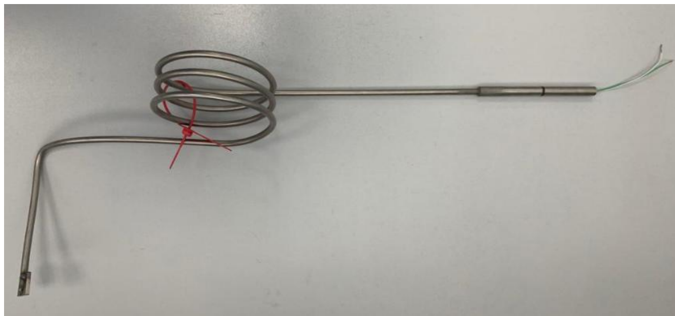
Рисунок 1 – Общий вид ТП
