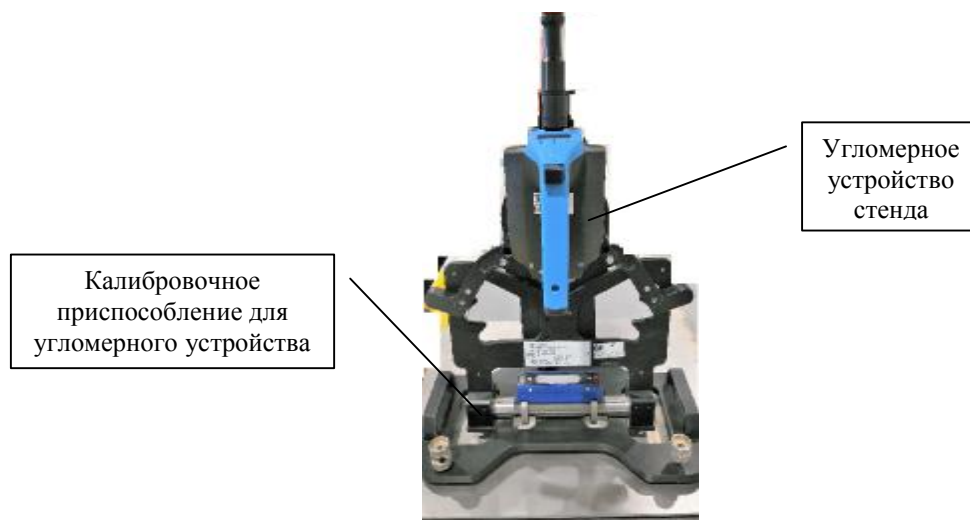
Рисунок 2 - Устройство угломерное с калибровочным приспособлением
