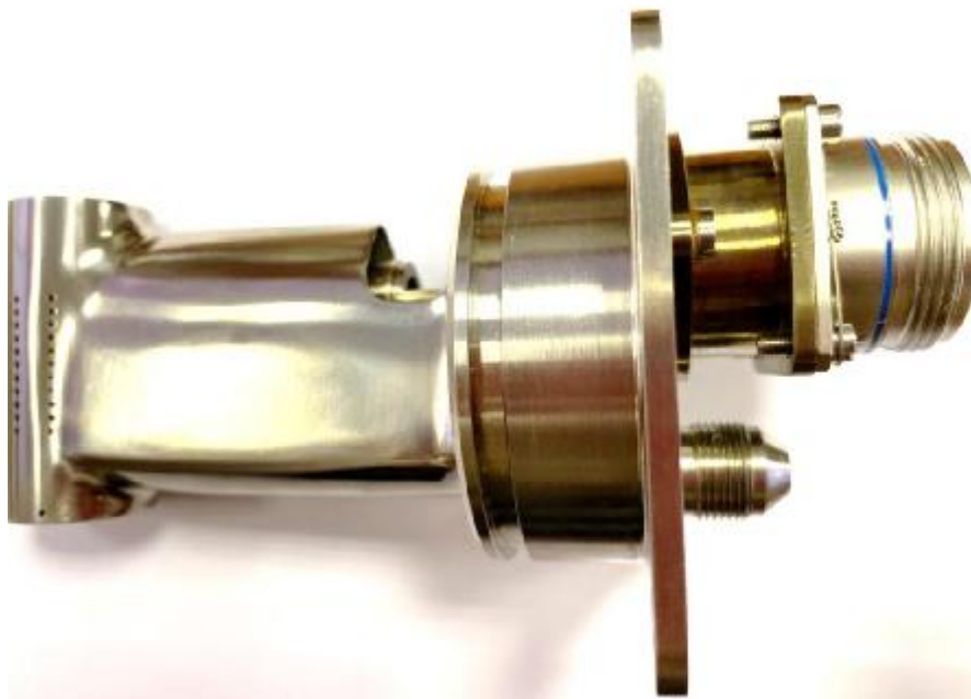
Рисунок 1 – Общий вид датчиков
