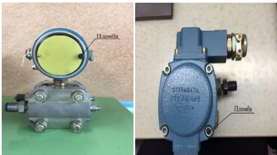
Рисунок 3 - Место нанесения пломбы
