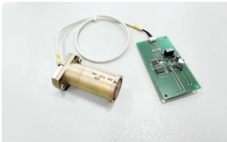
Рисунок 4 – Внешний вид измерителей угла наклона двухкоординатных ИИ-Д3а в бескорпусном исполнении
