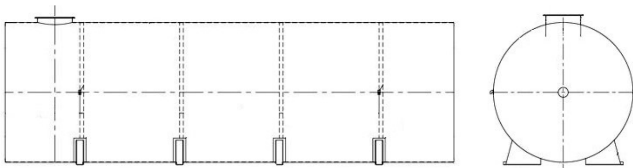
Рисунок 1 – Эскиз общего вида резервуаров стальных горизонтальных цилиндрических РГС-25
