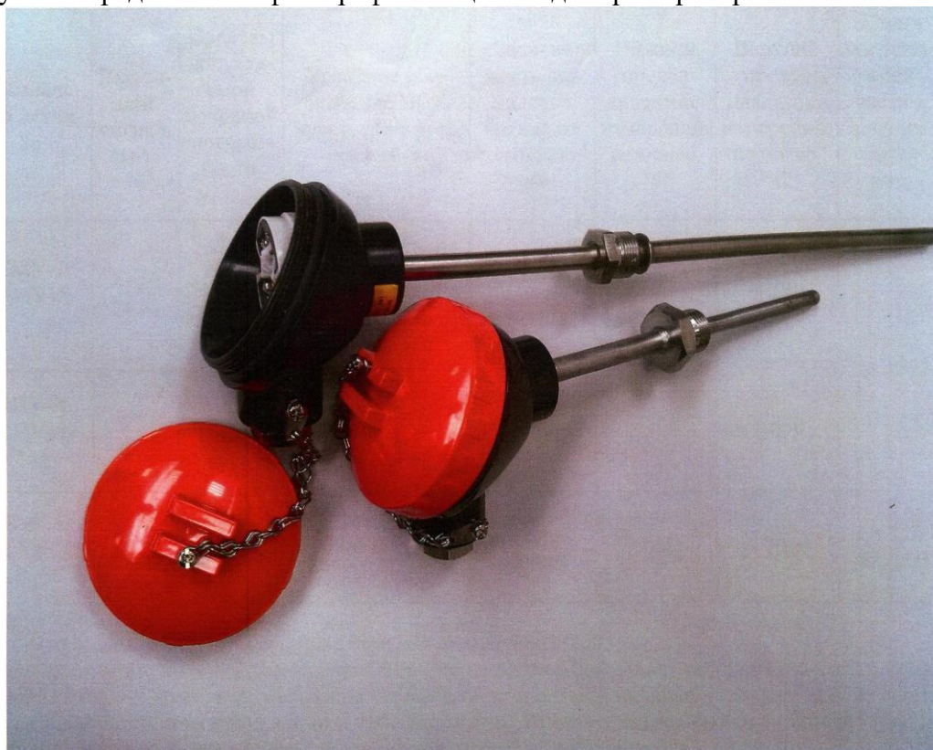
Рисунок 1 – Общий вид термопреобразователей с унифицированным выходным сигналом ТСМУ-Л, ТСПУ-Л, ТХАУ-Л, ТСМУ-Л-Ех, ТСПУ-Л-Ех, ТХАУ-Л-Ех Пломбирование термопреобразователей не предусмотрено.
