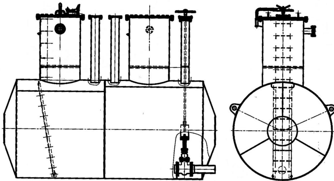
Рисунок 1 – Общий вид эскиза резервуара РГС-12,5
