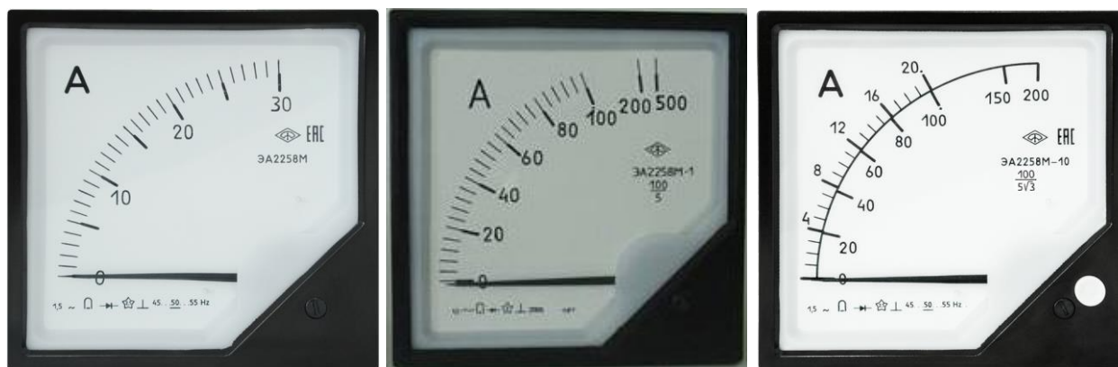
Рисунок 1 – Общий вид приборов ЭА2258М, ЭА2258М-1, ЭА2258М-10
