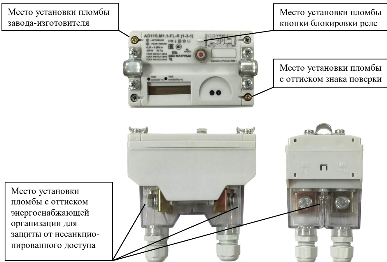
Рисунок 2 – Общий вид счетчика в корпусе AD11S.M1 и схема его пломбировки
