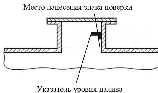
Рисунок 3 – Схема пломбировки от несанкционированного изменения положения уровня налива, обозначение места нанесения знака поверки
